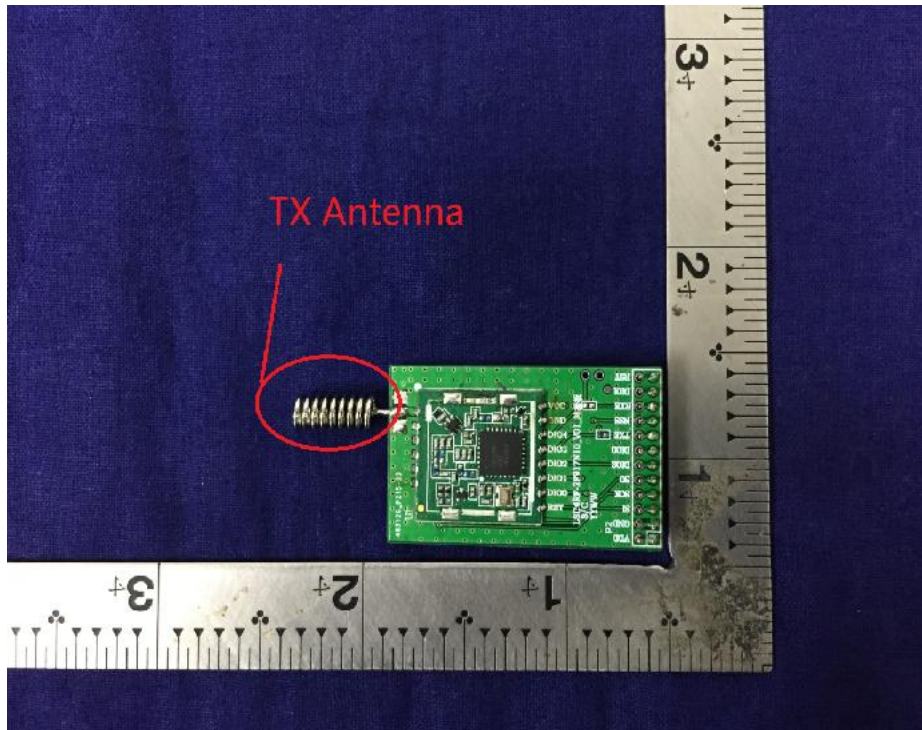
(3) EUT Photo
