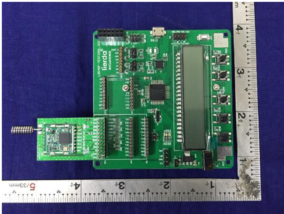
(5) EUT Photo
