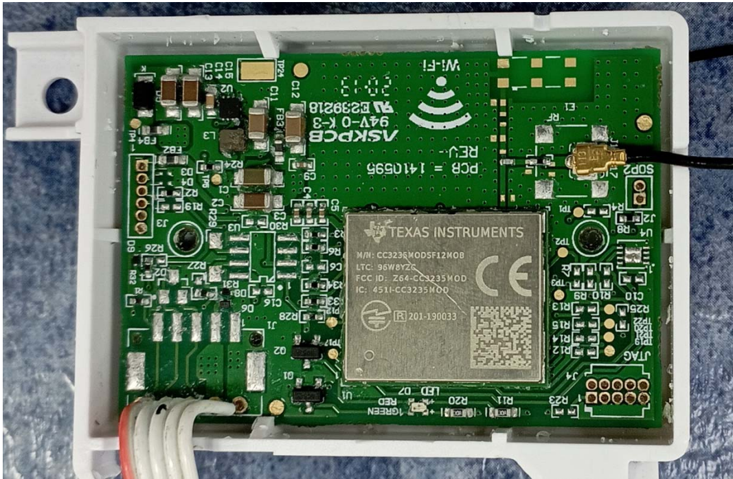
WiFi Module Antenna
