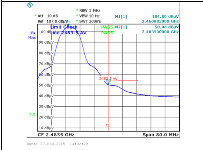
Band Edge, Right Side (Average) - 802.11b (EMW3165-E)
