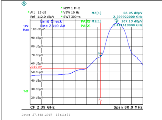
Band Edge, Left Side (Average) - 802.11b (EMW3165-E)
