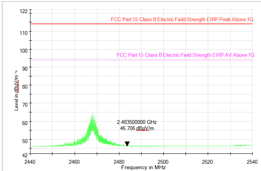
Electric Field Strength 1-18GdBuV TXEIRP
