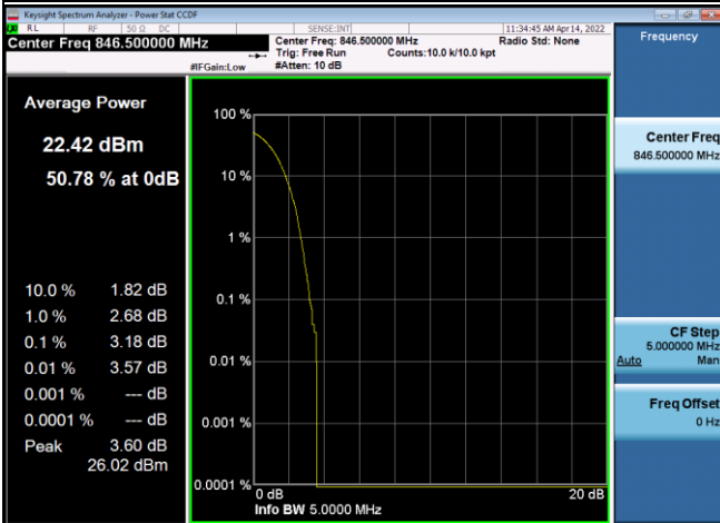
QPSK-20625
