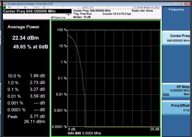
16QAM-20625
