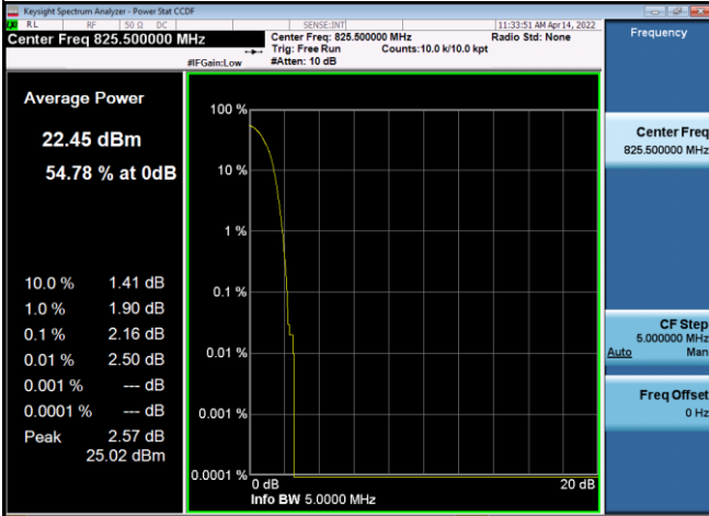
QPSK-20415
