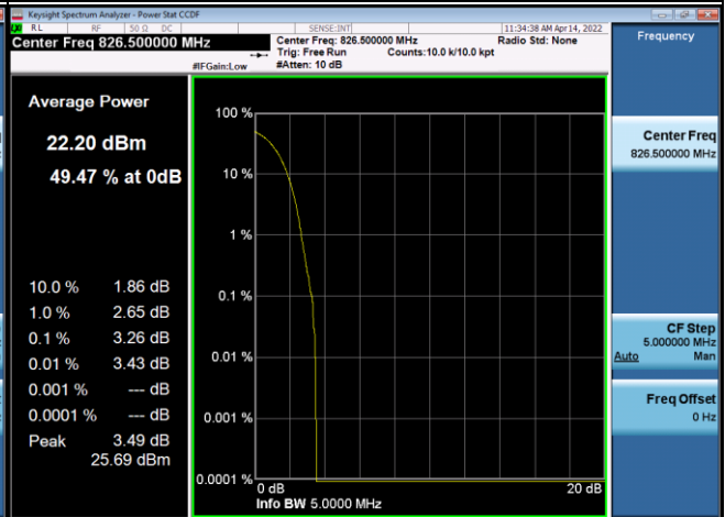
16QAM-20425
