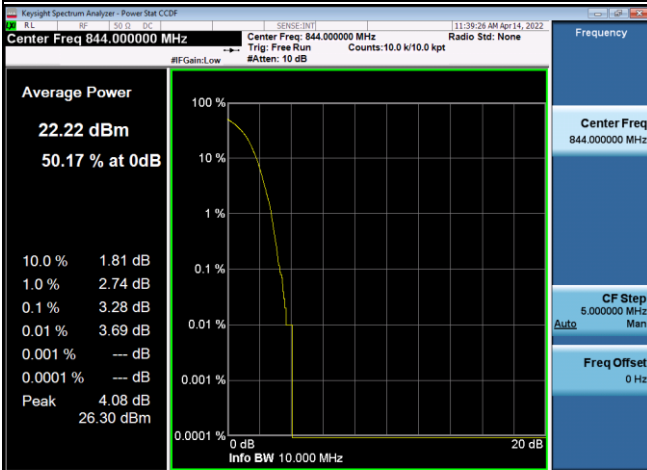
QPSK-20600
