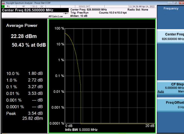
QPSK-20425
