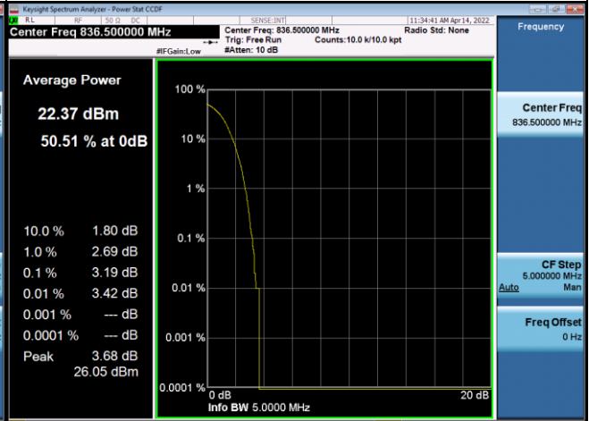
QPSK-20525
