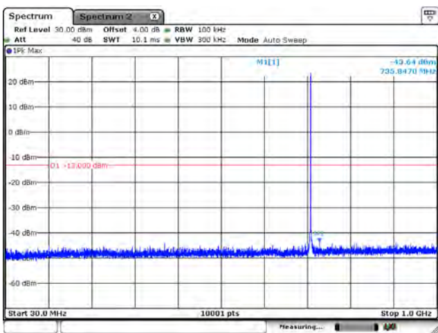
CH23178_15k_QPSK_1RB0_Below 1G
