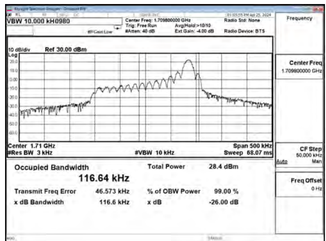
QPSK_CH133120_15k_1RB11
