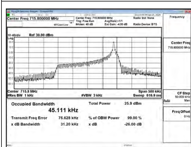
BPSK_CH134180_3.75k_1RB47
