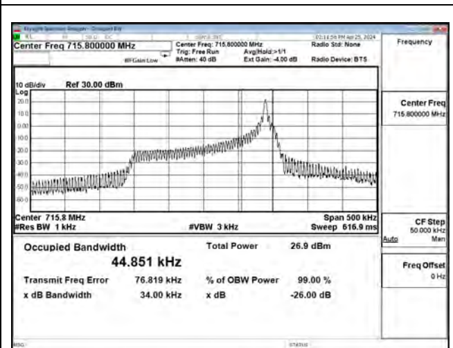
QPSK_CH134180_3.75k_1RB47
