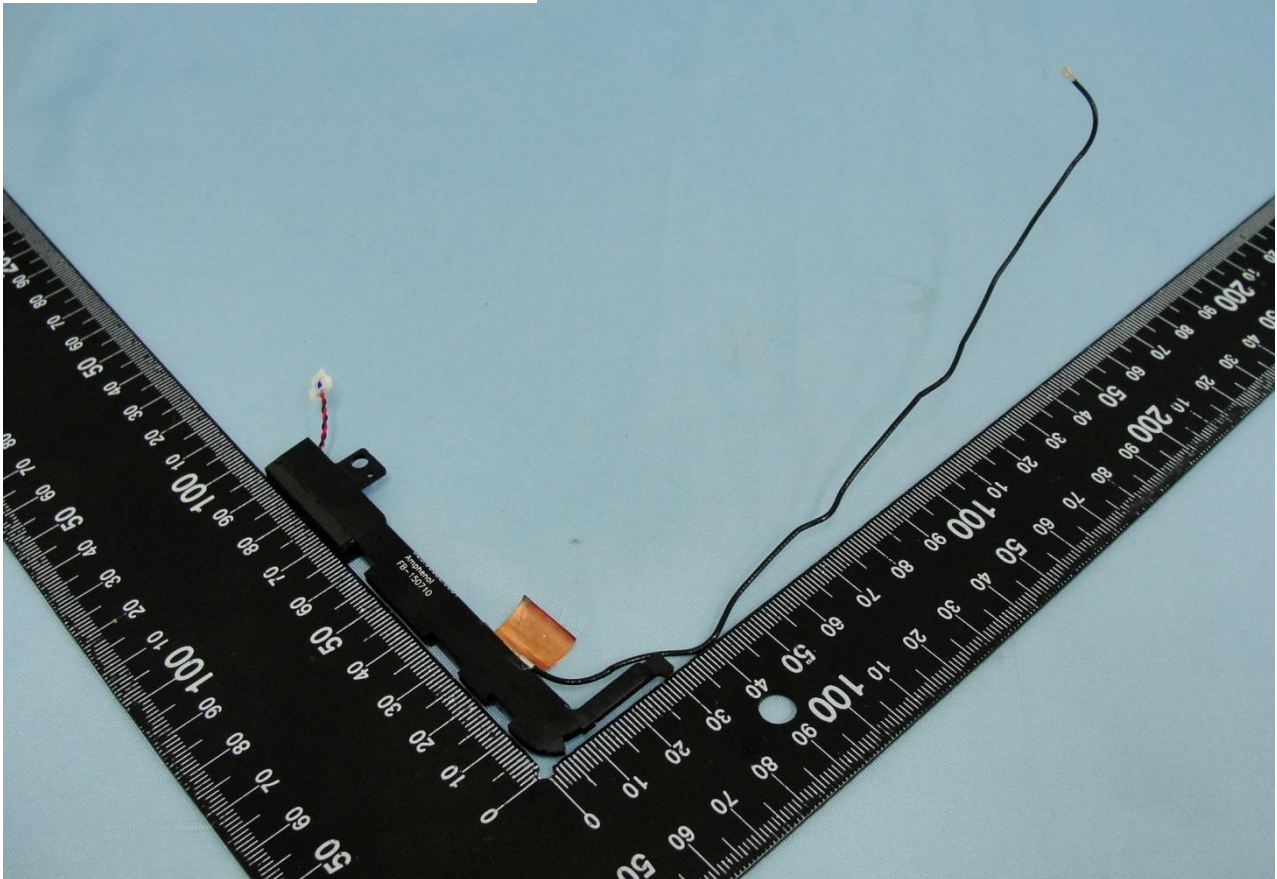
GPS Antenna & WWAN Aux. Antenna
