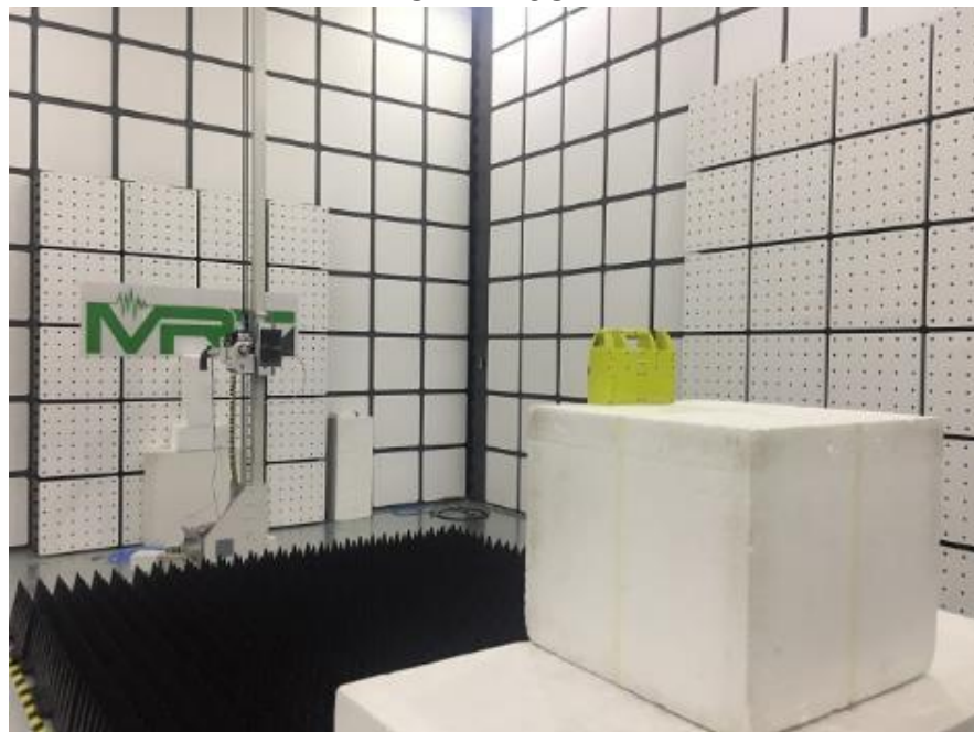
1GHz ~ 18GHz
