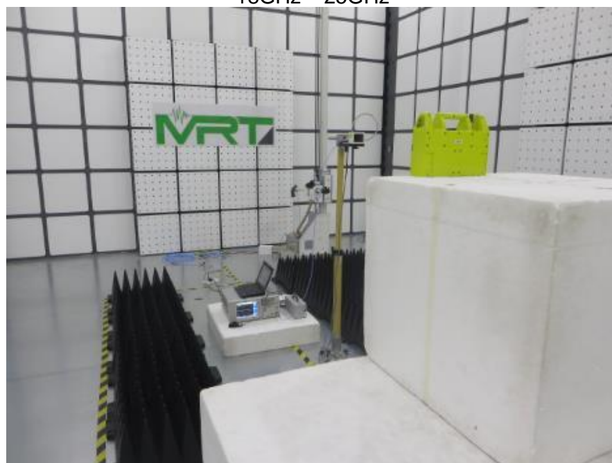
18GHz ~ 25GHz
