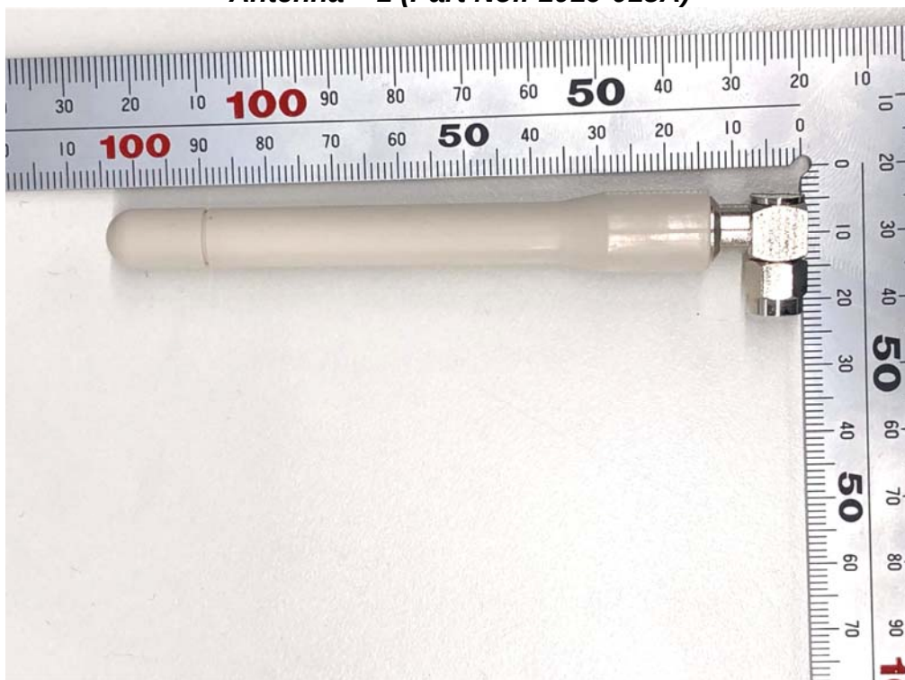
Antenna – 1 (Part No.: 1019-015A)
