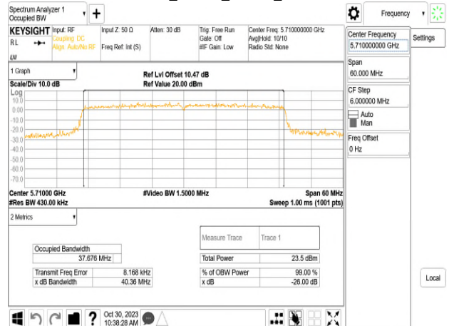
802.11ax_40MHz_Chain1_5710MHz
