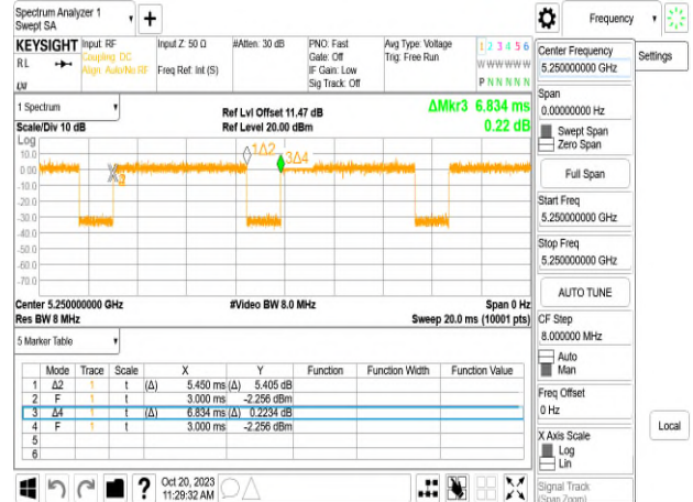
802.11ax_160MHz_Chain0_5250MHz
