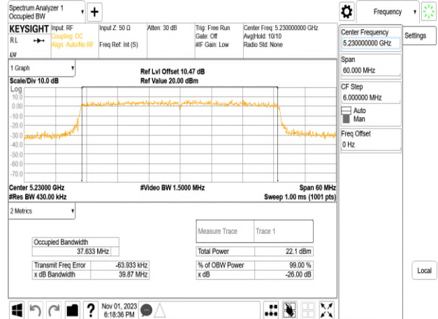
802.11ax_40MHz_Chain1_5230MHz
