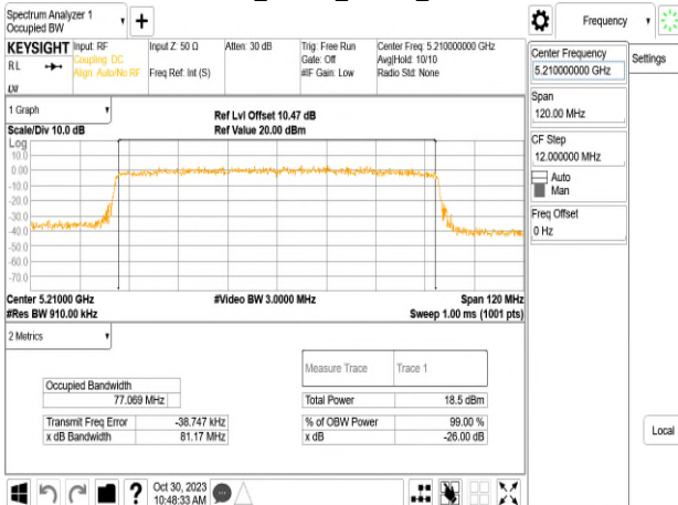
802.11ax_80MHz_Chain1_5210MHz
