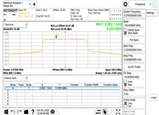
802.11ax_40MHz_Chain1_5270MHz
