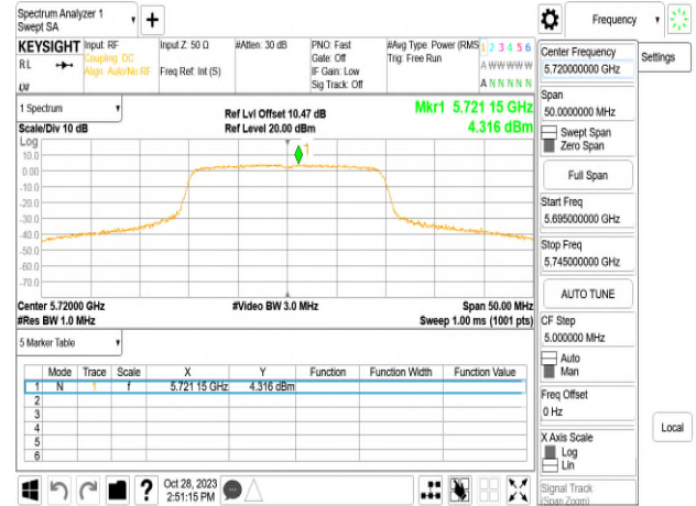
802.11ax_20MHz_Chain0_5720MHz_UNII 3
