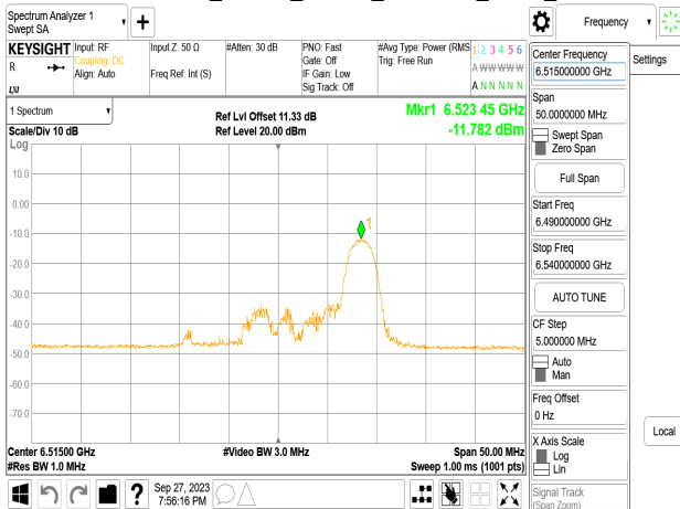
802.11ax_20MHz_Chain1_6515MHz_RU52_40
