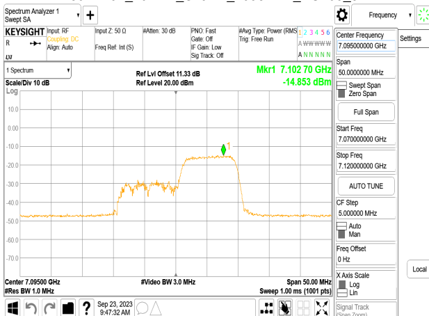
802.11ax_20MHz_Chain1_7095MHz_RU26_8
