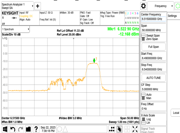
802.11ax_20MHz_Chain1_6515MHz_RU52_40
