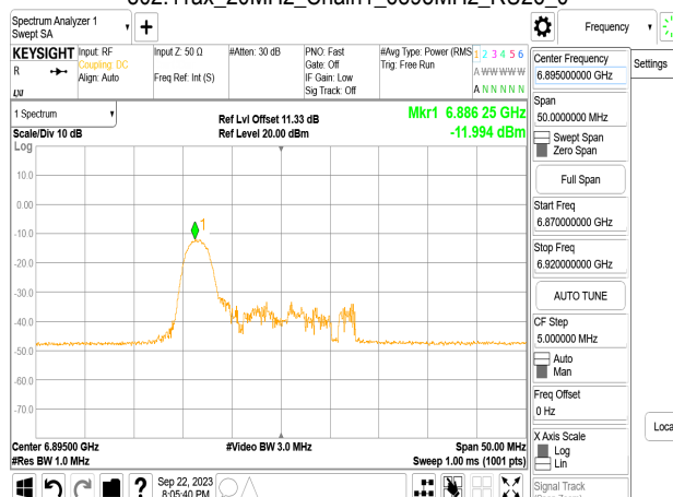
802.11ax_20MHz_Chain1_6895MHz_RU52_37
