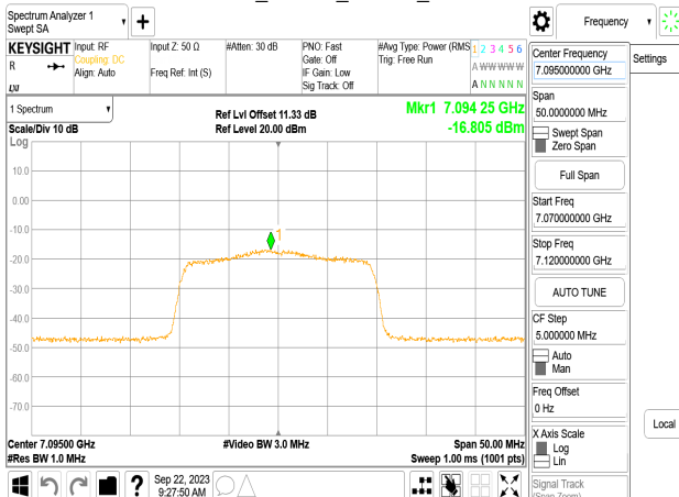
802.11ax_20MHz_Chain1_7095MHz_RU106_54
