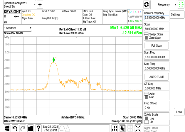
802.11ax_20MHz_Chain1_6535MHz_RU26_0
