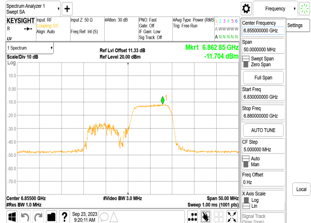
802.11ax_20MHz_Chain1_6855MHz_RU26_8
