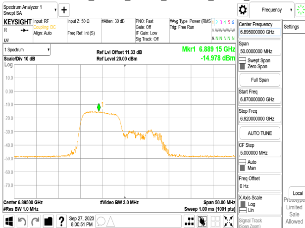
802.11ax_20MHz_Chain0_6895MHz_RU26_0
