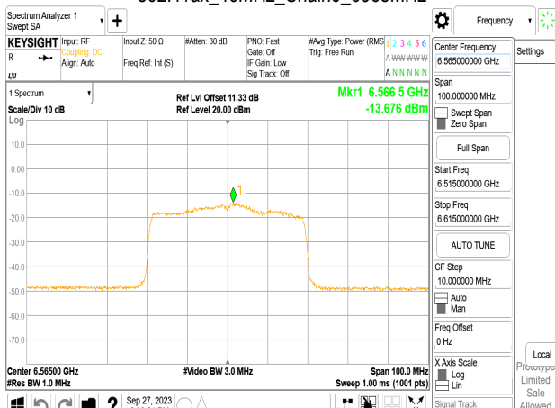
802.11ax_40MHz_Chain0_6565MHz
