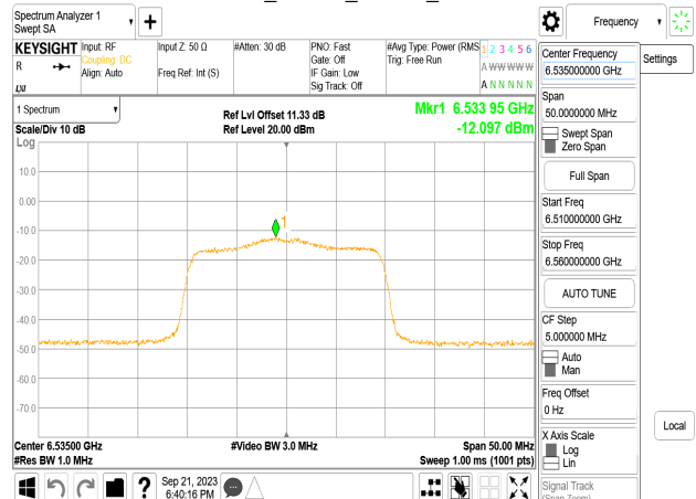
802.11ax_20MHz_Chain1_6535MHz_RU106_53
