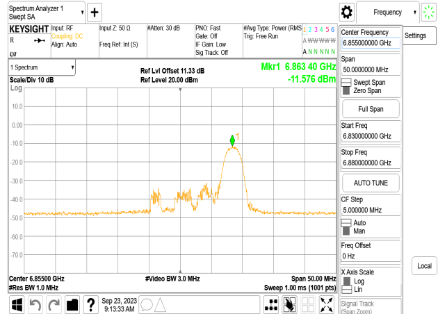
802.11ax_20MHz_Chain1_6855MHz_RU52_40
