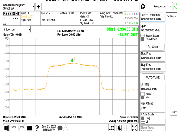
802.11ax_20MHz_Chain1_6995MHz
