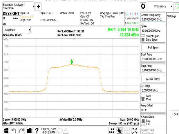
802.11ax_20MHz_Chain1_5955MHz_RU106_53
