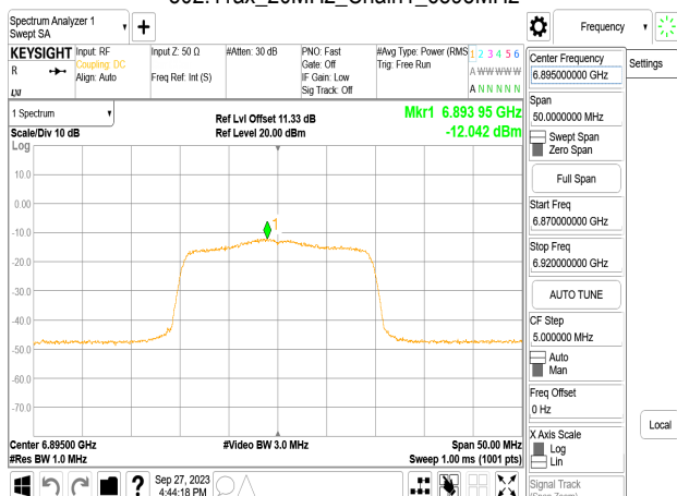
802.11ax_20MHz_Chain1_6895MHz_RU106_53
