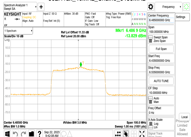
802.11ax_40MHz_Chain0_6485MHz
