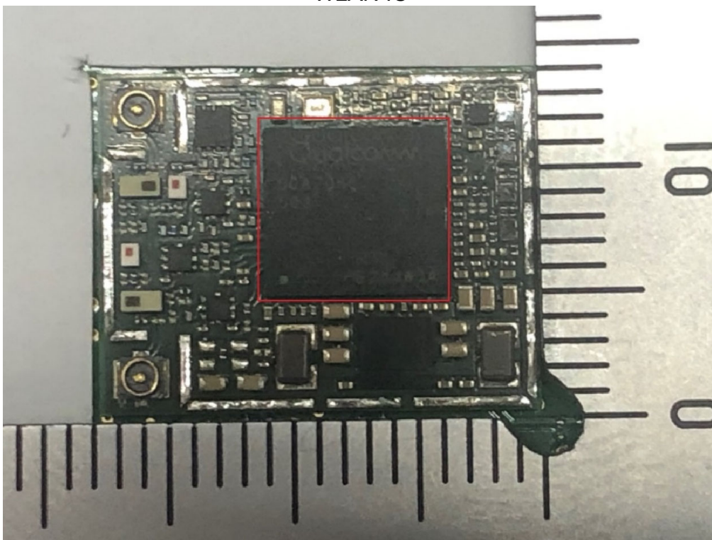
WLAN IC
