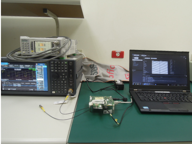
FCC_15_407_WLAN_6E_Normal_CBP_Setup
