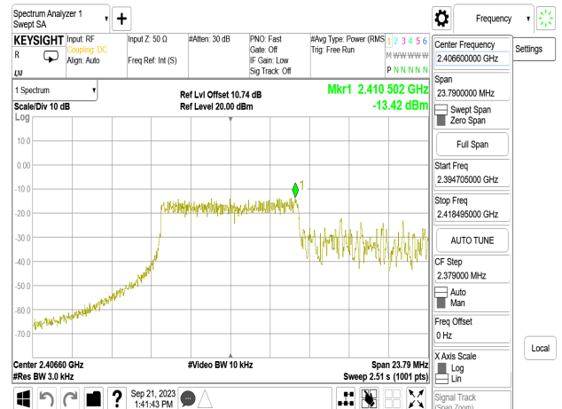
802.11ax_20MHz_Chain1_2412MHz_RU26_0
