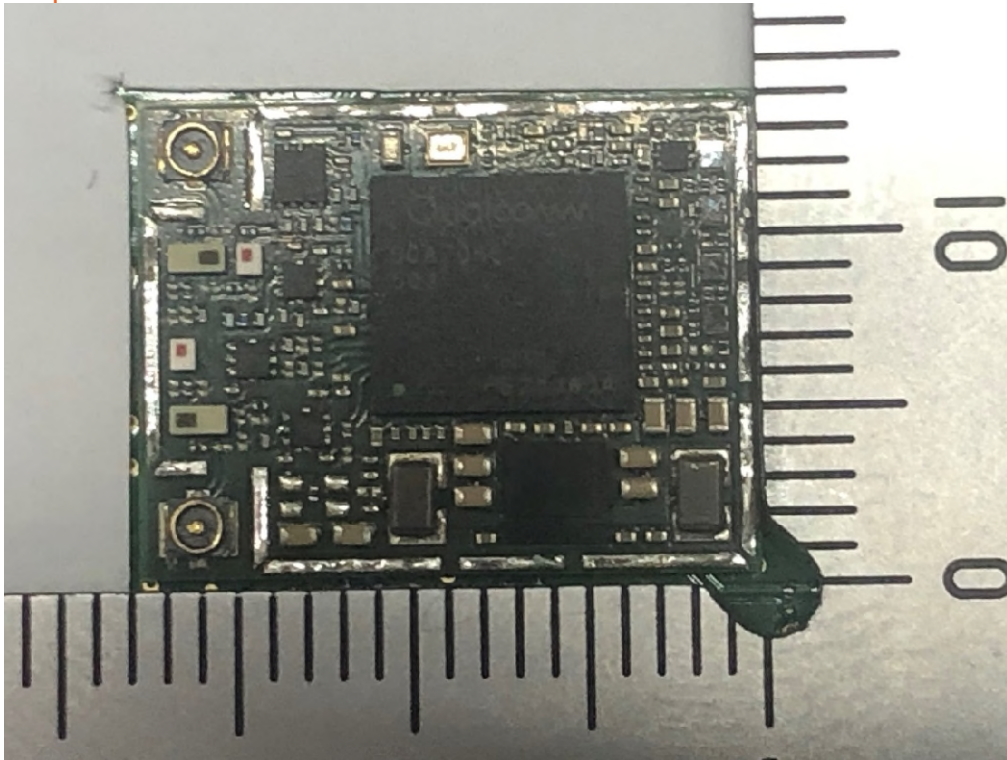
WLAN IC
