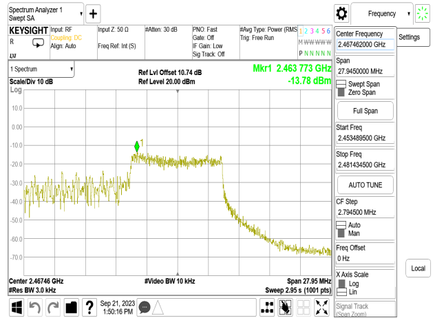
802.11ax_20MHz_Chain1_2462MHz_RU26_8
