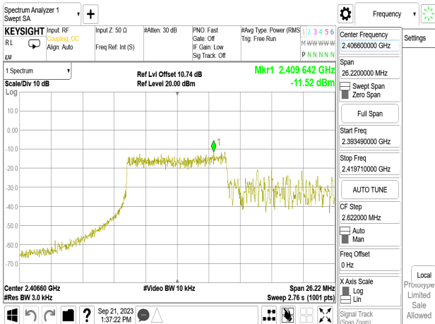
802.11ax_20MHz_Chain0_2412MHz_RU26_0
