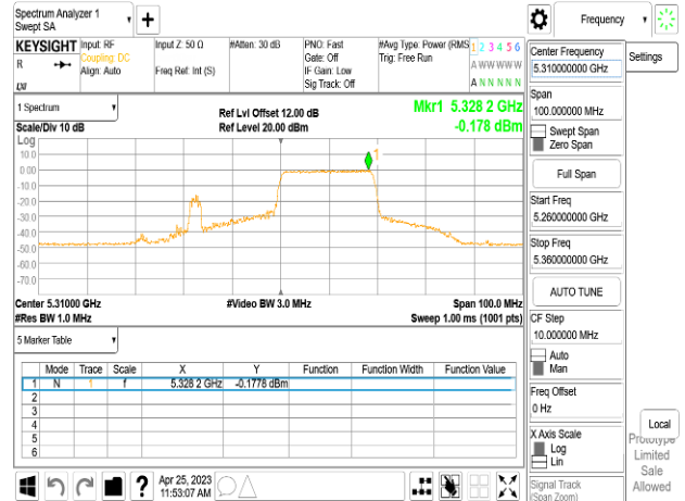
802.11ax_40MHz_Chain1_5310MHz_RU242_62
