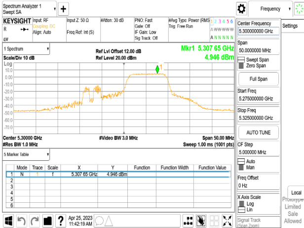
802.11ax_20MHz_Chain1_5300MHz_RU26_8
