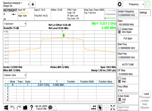
802.11ax_40MHz_Chain0_5230MHz_RU242_61
