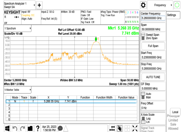
802.11ax_20MHz_Chain1_5260MHz_RU52_40
