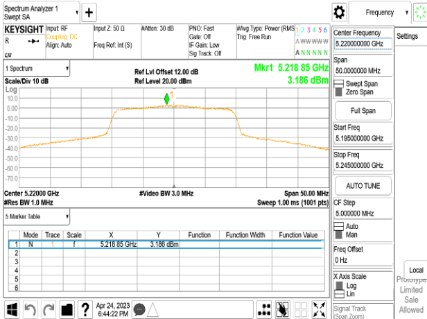
802.11ax_20MHz_Chain1_5220MHz_RU106_53
