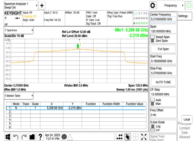
802.11ax_80MHz_Chain1_5210MHz_RU484_65
