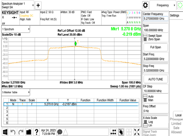
802.11ax_40MHz_Chain0_5270MHz_RU242_62
