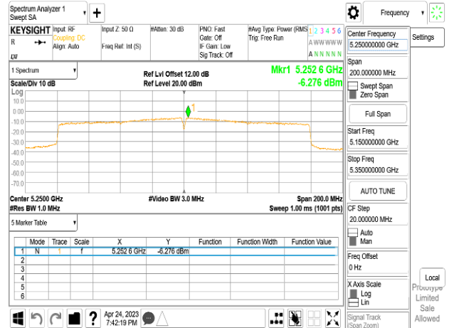
802.11ax_160MHz_Chain1_5250MHz
