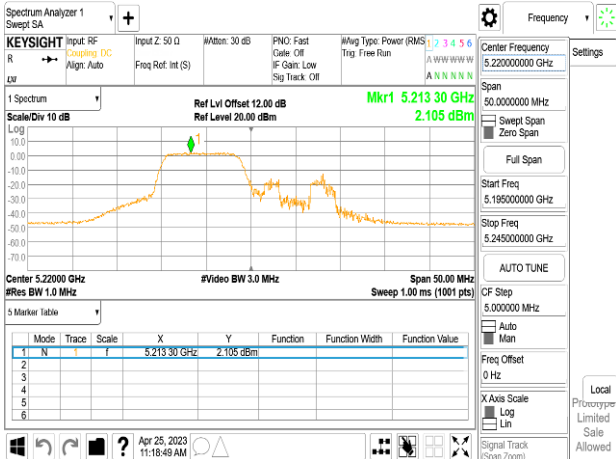
802.11ax_20MHz_Chain1_5220MHz_RU26_0
