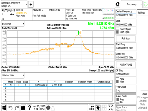
802.11ax_20MHz_Chain1_5320MHz_RU52_40
