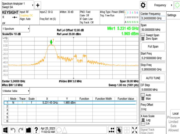
802.11ax_20MHz_Chain1_5240MHz_RU52_37
