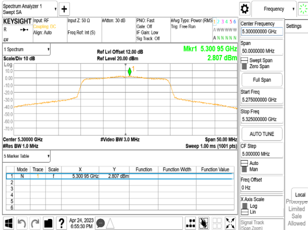
802.11ax_20MHz_Chain1_5300MHz_RU106_54
