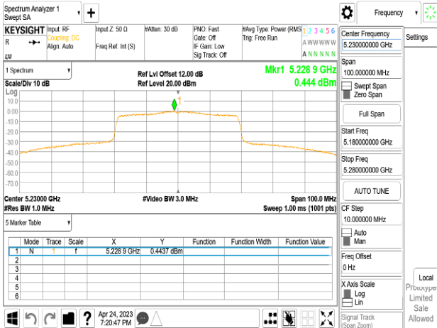
802.11ax_40MHz_Chain1_5230MHz_RU242_61
