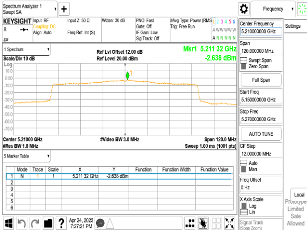
802.11ax_80MHz_Chain0_5210MHz_RU484_65
