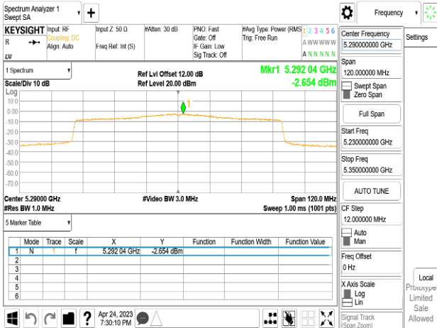
802.11ax_80MHz_Chain1_5290MHz_RU484_66
