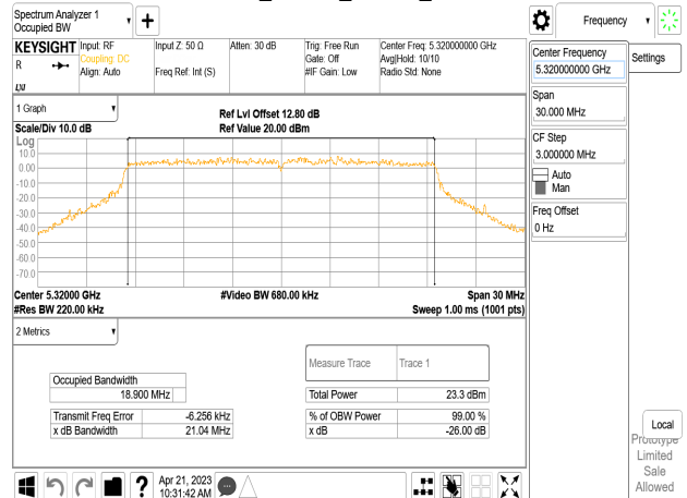
802.11ax_20MHz_Chain0_5320MHz
