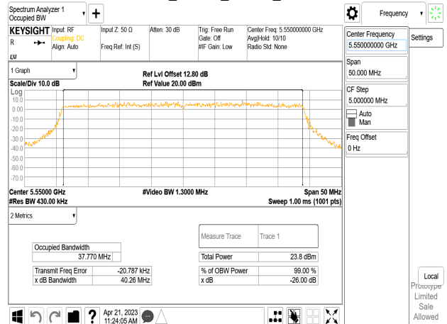
802.11ax_40MHz_Chain1_5550MHz
