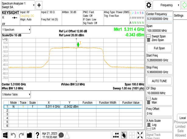
802.11ax_40MHz_Chain1_5310MHz
