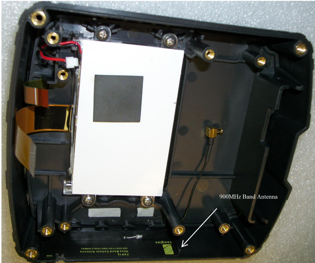
EUT 900MHz Band Antenna
