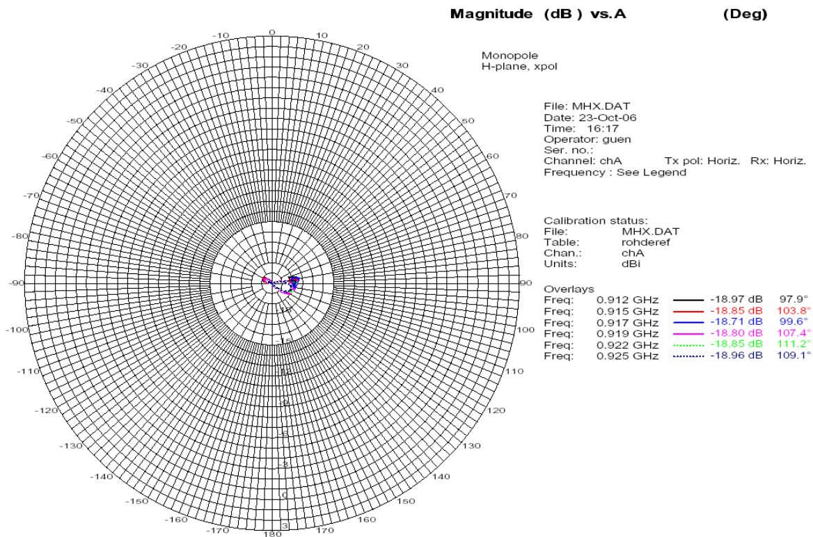
Fig 8: Monopole, H-plane, xpol (horizontal pol)
