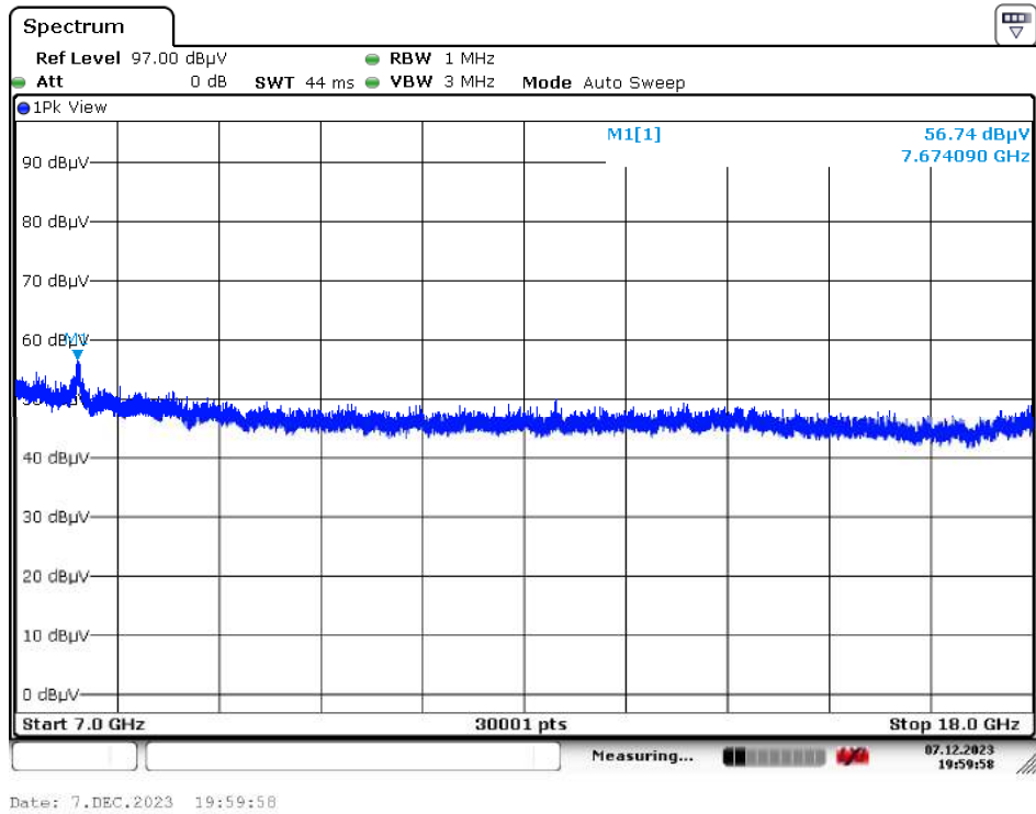
Downlink / 5G NR 100 MHz / AC
