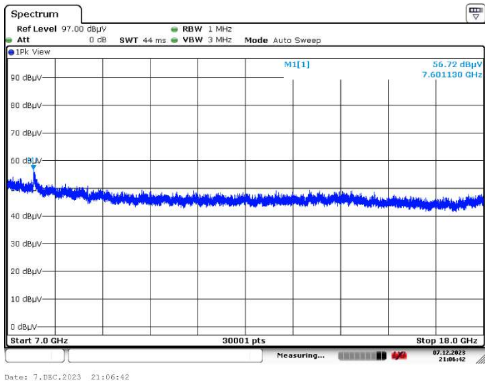
Downlink / 5G NR 100 MHz / DC
