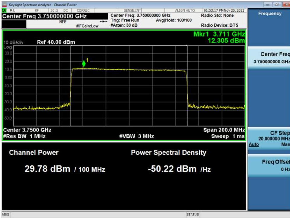
PSD / 3.7 GHz Service / Uplink / 5G NR 100 MHz
