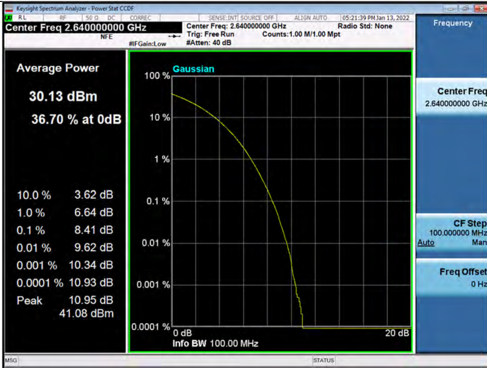
PAPR / BRS/EBS / Uplink / 5G NR 100 MHz
