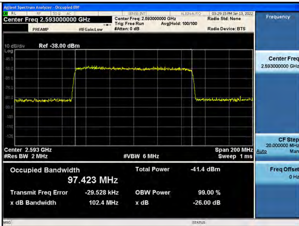
Input / BRS/EBS / Uplink/ 5G NR 100 MHz
