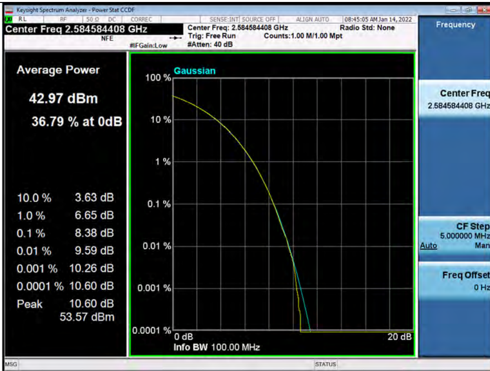
PAPR / BRS/EBS / Downlink / 5G NR 100 MHz
