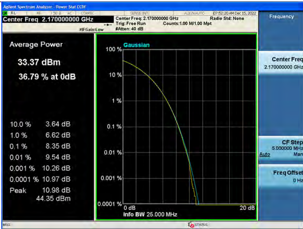
PAPR / AWS / Downlink / 5G NR 20 MHz
