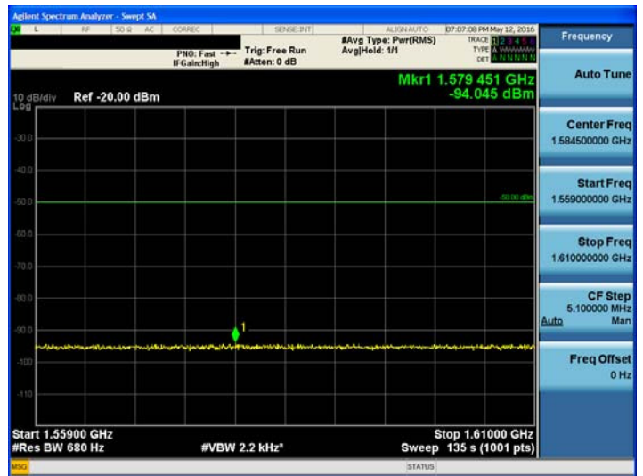
1559MHz ~ 1610MHz
