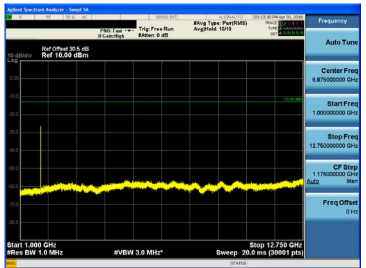
1GHz ~ 12.75GHz
