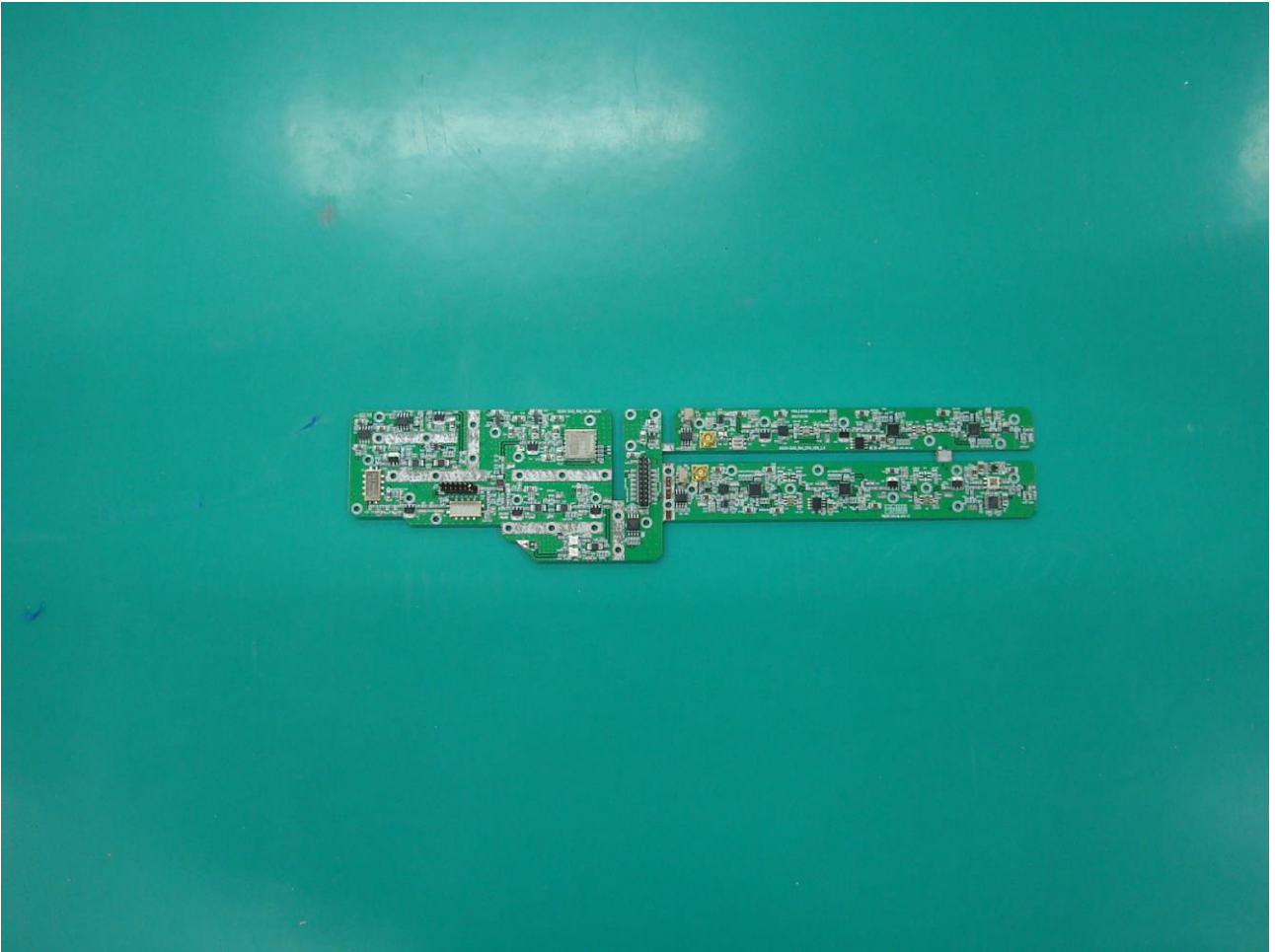
MODULE-TOP
