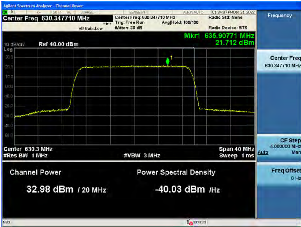
PSD / 600 MHz Service / Downlink / 5G NR 20 MHz
