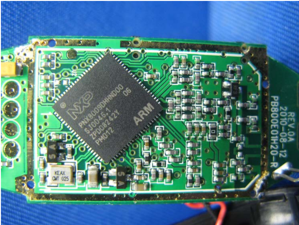
Headset RF Module
