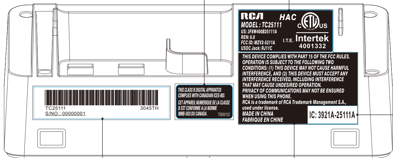
SERIAL NO. LABEL, GZ PRINT, SIZE: 60*14 mm TF表示广州生产, TH表示惠州生产
