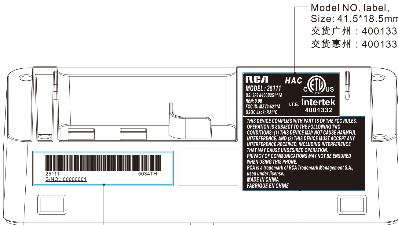
SERIAL NO.LABEL, GZ PRINT, SIZE: 60*14 mm TF表示广州生产, TH表示惠州生产
