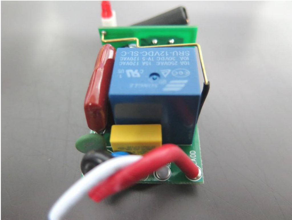
InPho3-MainBoard
