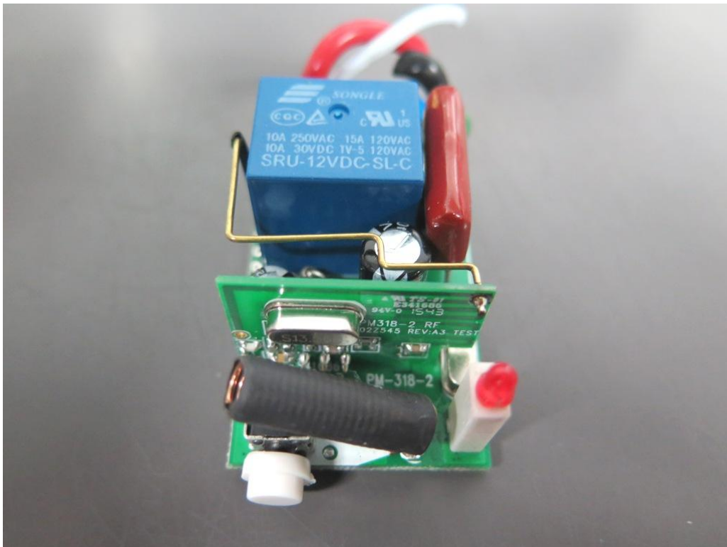
InPho2-MainBoard
