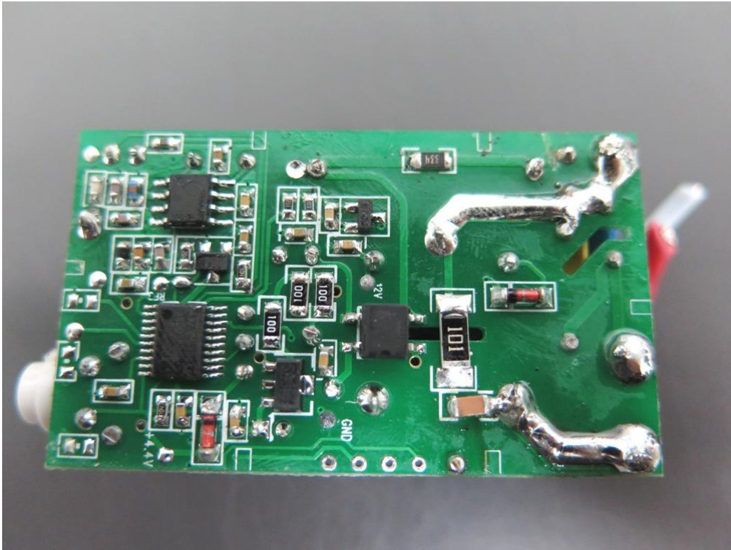
InPho5-MainBoard
