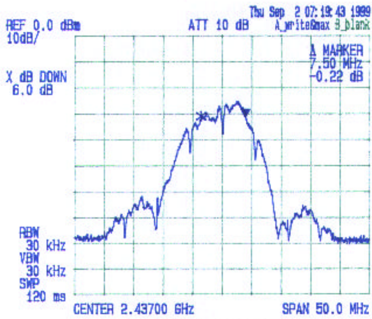
2 Mbps DQPSK
