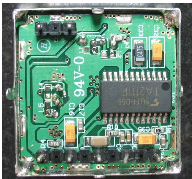
UHF module
