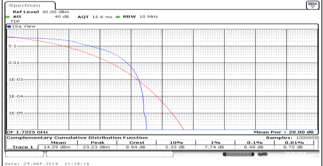
Band4_20MHz_QPSK_20175_6
