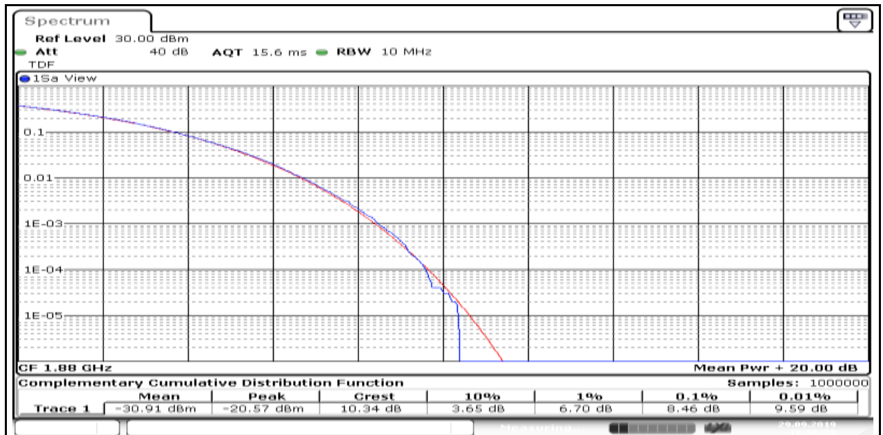
Band2_15MHz_QPSK_18900_6
