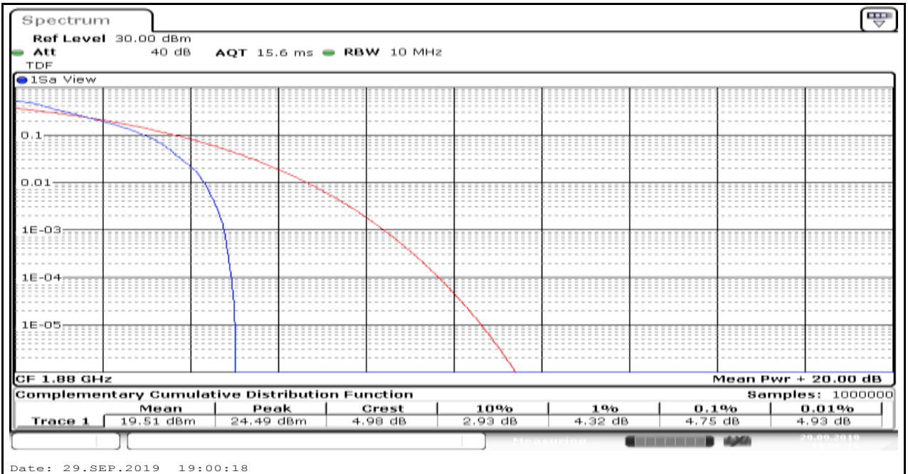
Band2_20MHz_QPSK_18900_6
