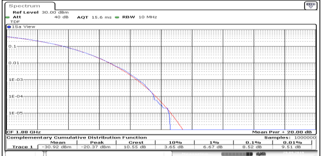
Band2_15MHz_QPSK_18900_6
