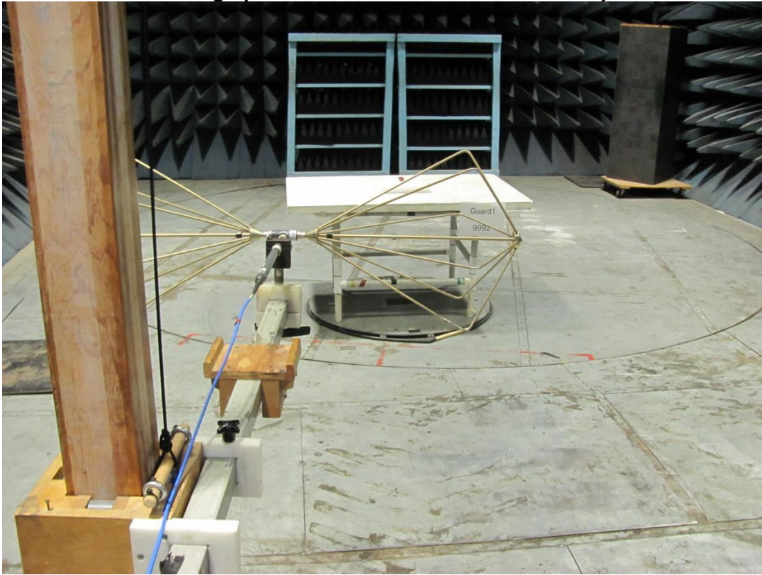
30-200 MHz
