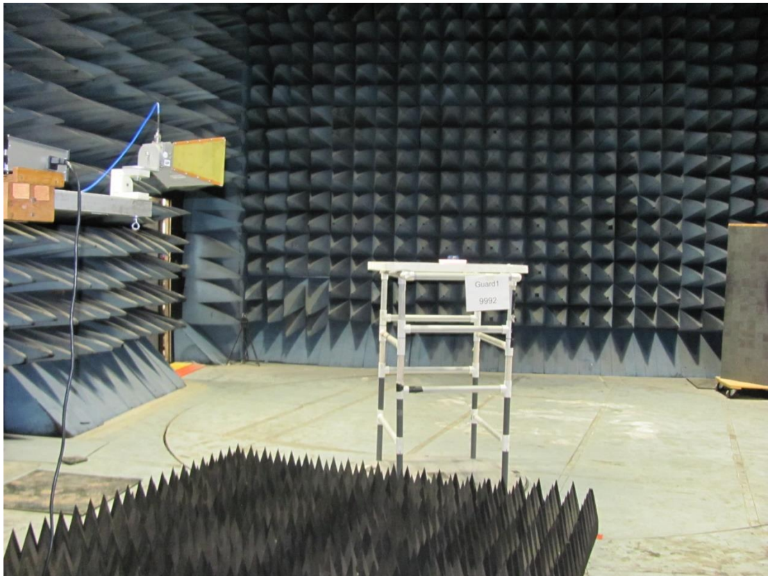
1-18 GHz
