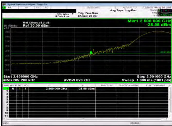
Band Edge_Band7 15MHz_QPSK 1 0_LowCH20825-2507.5
