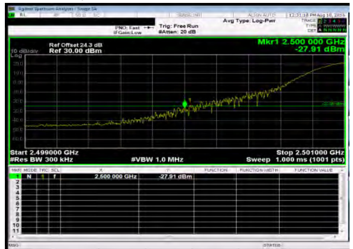
Band Edge_Band7 20MHz_QPSK 1 0_LowCH20850-2510
