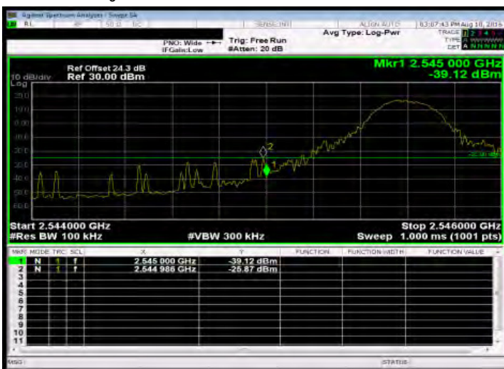
Band Edge_Band41 10MHz_QPSK 1 0_LowCH40190-2550
