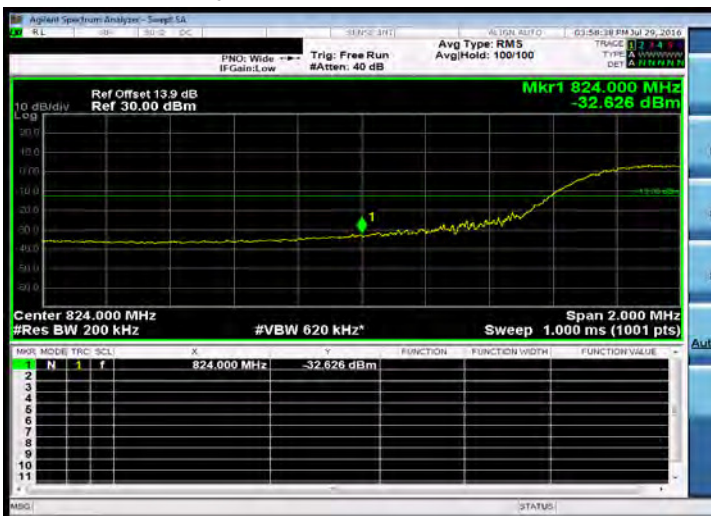
Band Edge_Band26 10MHz_QPSK 75 0_Low
