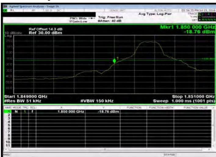
Band Edge_Band2 5MHz_QPSK 1 0_LowCH18625-1852.5
