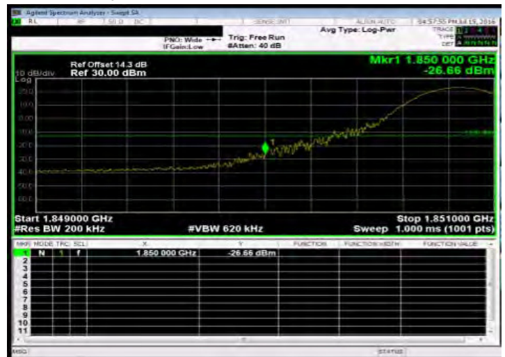
Band Edge_Band2 15MHz_QPSK 1 0_LowCH18675-1857.5
