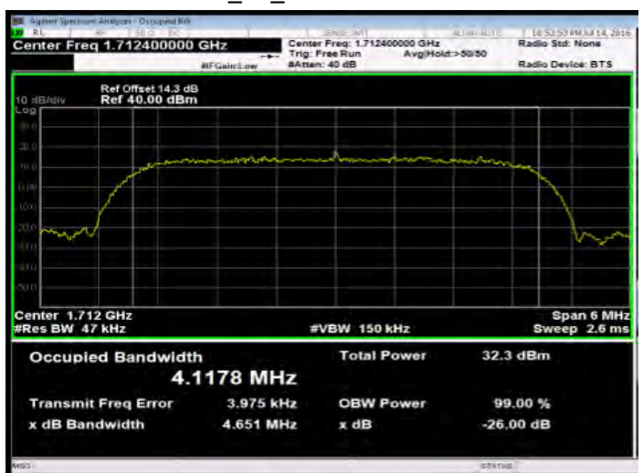
HSUPA_B4_LowCH1312-1712.4
