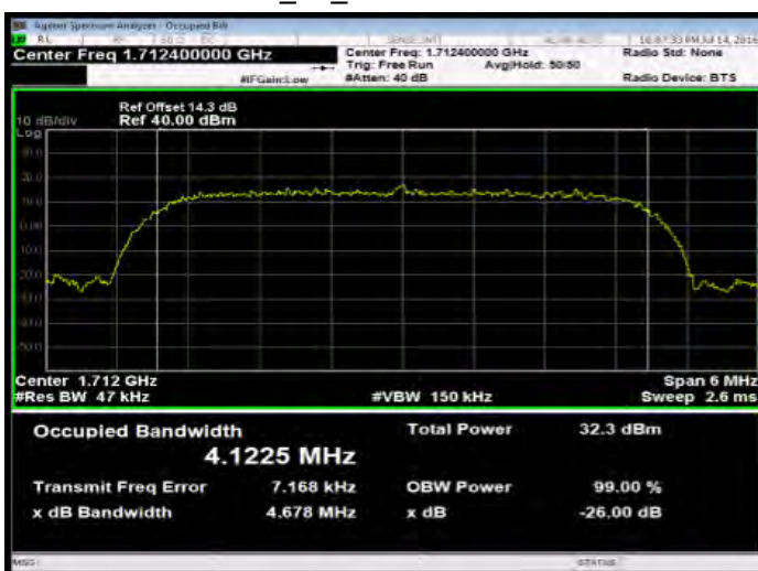
WCDMA_B4_LowCH1312-1712.4
