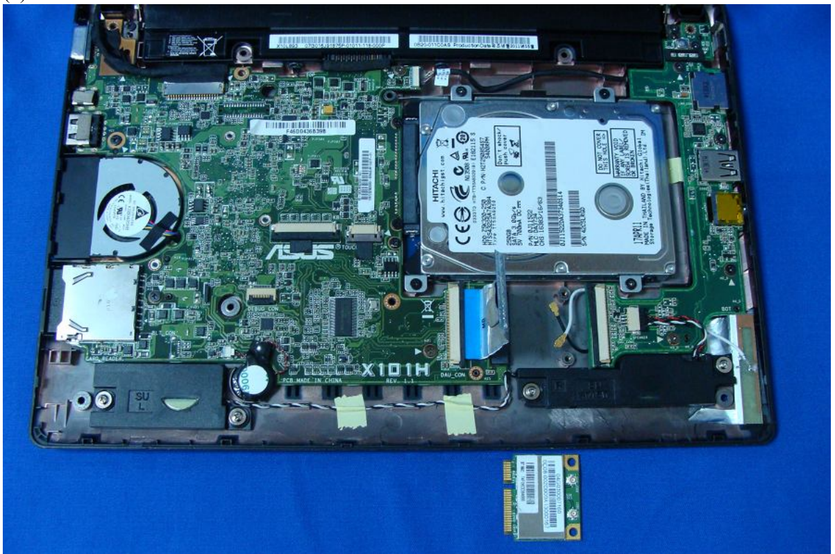
(8) EUT Photo
