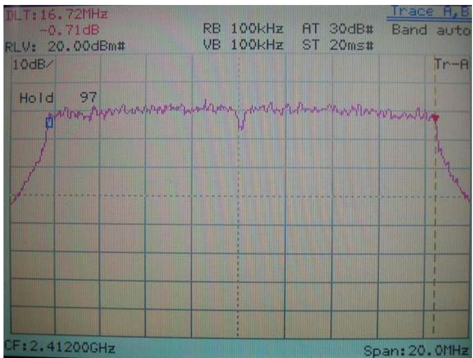
IEEE 802.11g
