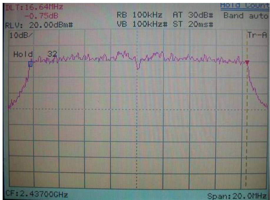
IEEE 802.11g
