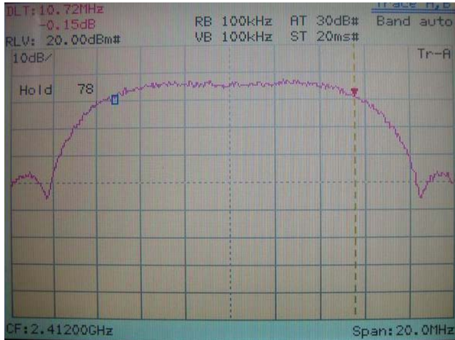
IEEE 802.11b
