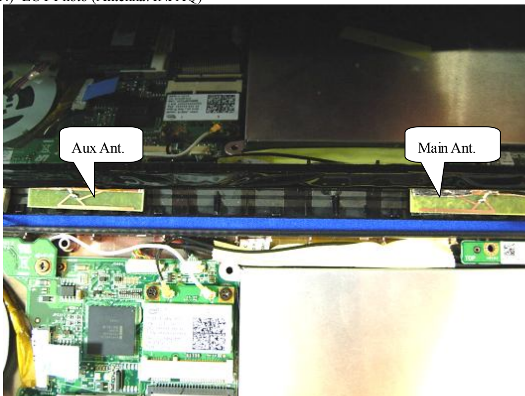
(24) EUT Photo (Antenna: INPAQ)
