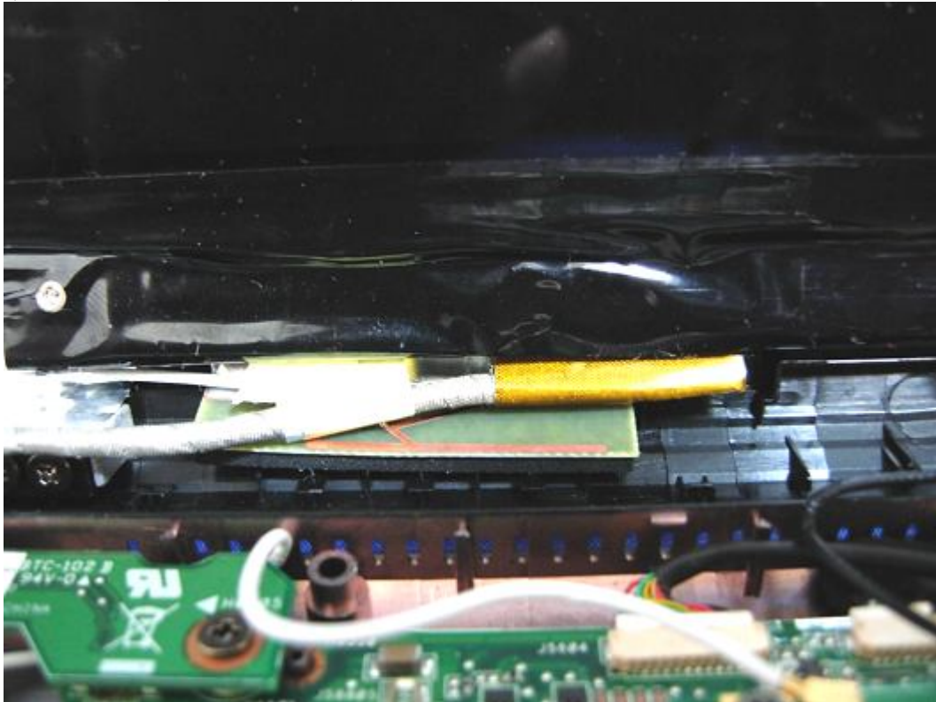
(26) EUT Photo (Antenna: INPAQ)
