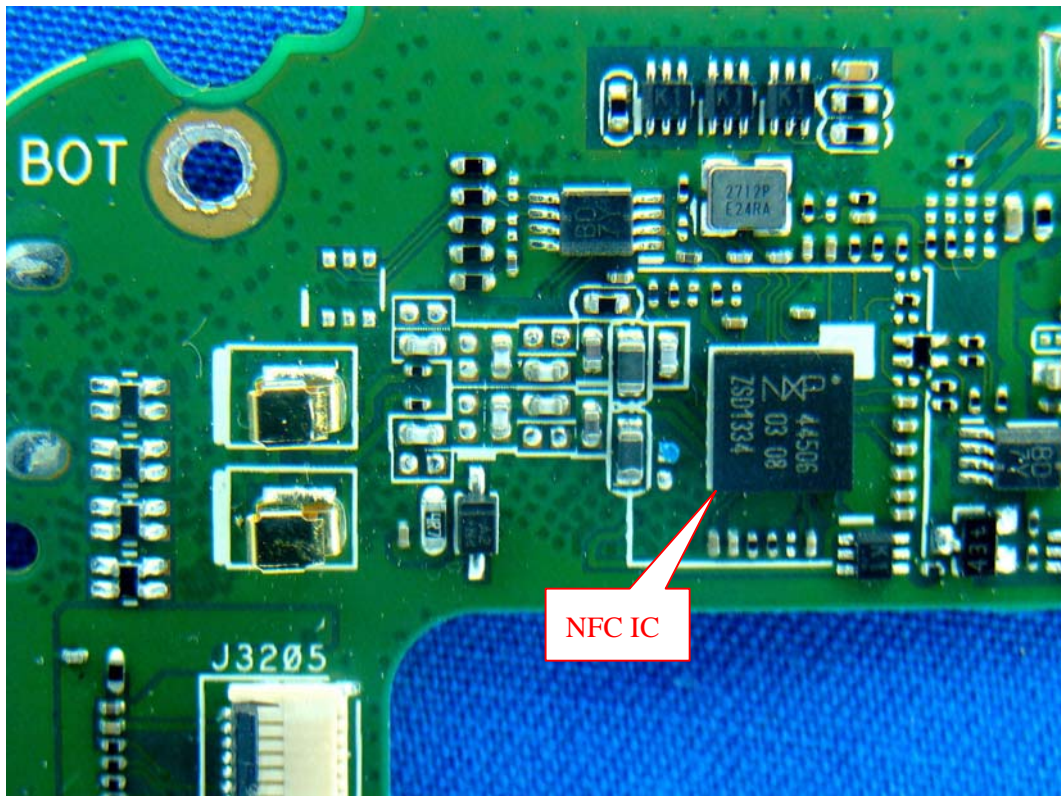
(32) EUT Photo (NFC)
