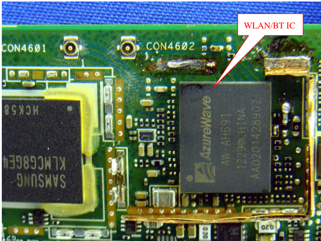
(31) EUT Photo (WLAN+BT)
