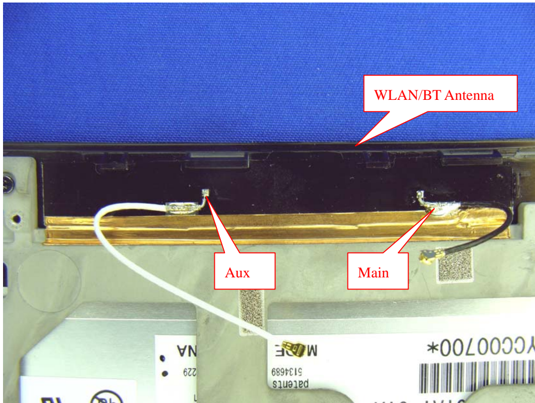
(21) EUT Photo (WLAN+BT Ant)
