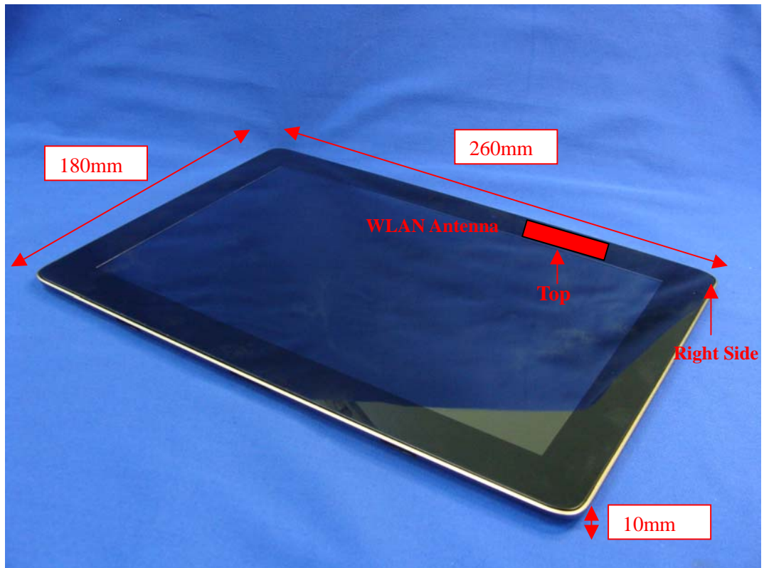
(2) EUT Photo
