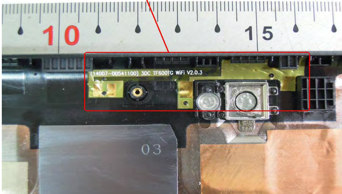
BT.WLAN antenna
