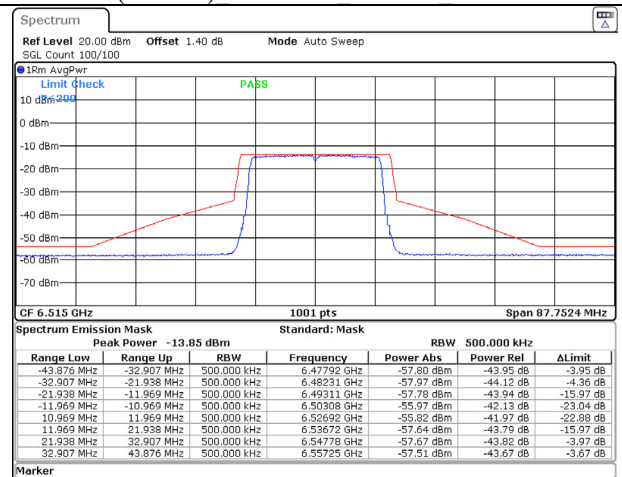
802.11ax (20MHz) 6515MHz Chain D NSS-1
