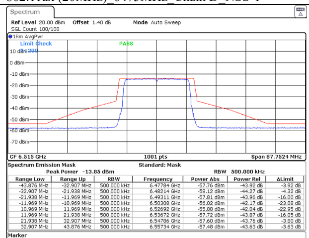
802.11ax (20MHz) 6515MHz Chain B NSS-1
