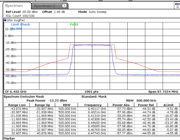
802.11ax (20MHz) 6435MHz Chain C NSS-1
