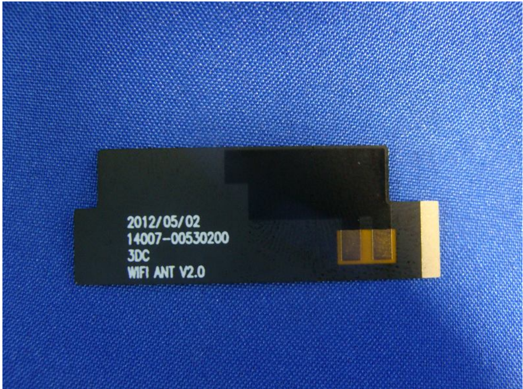
(24) EUT Photo - (Antenna: ACON)
