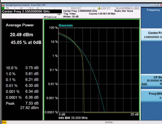
20MHz / 16QAM
